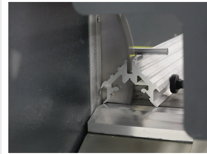
TT-405 Alüminyum için Çift Kafa Kesim Diagramı
