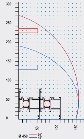
TT-405 Alüminyum için Çift Kafa Kesim Diagramı
